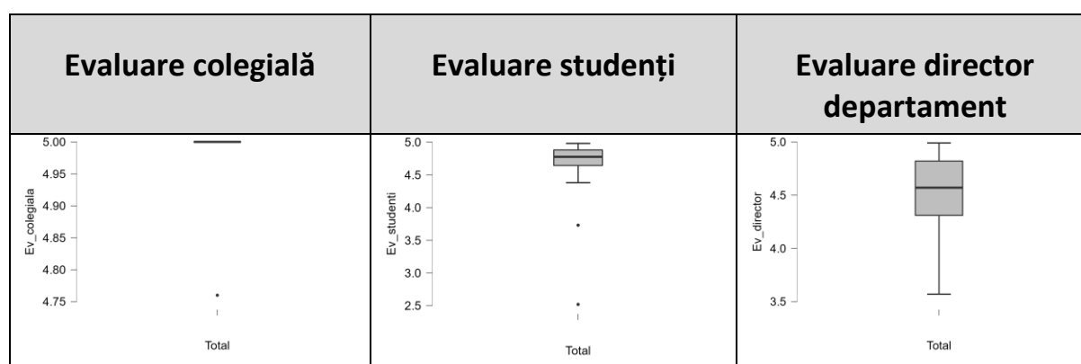
Figura 3. Diagrame boxplot aferente punctajelor obținute de cadrele didactice la evaluarea colegială, la evaluarea de către studenți, respectiv la evaluarea de către directorul de departament
