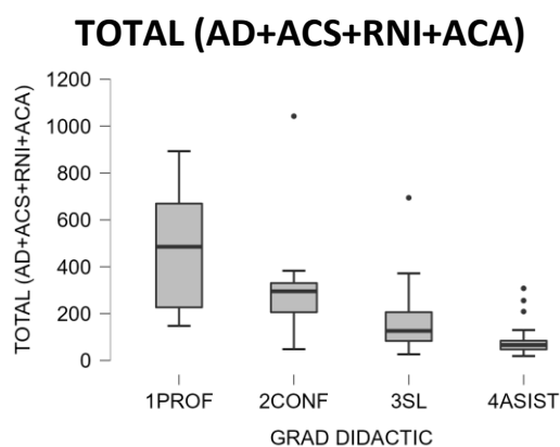
Figura 2. Diagrame boxplot aferentă punctajelor criteriilor din fișa de autoevaluare
