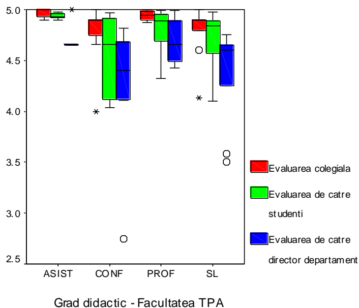
Figura 3 Diagrama boxplot aferentă punctajelor obținute de cadrele didactice la evaluarea colegială, la evaluarea de către studenți, respectiv la evaluarea de către directorul de departament
